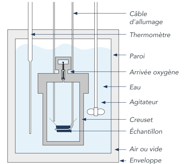
Bombe calorimétrique à oxygène
